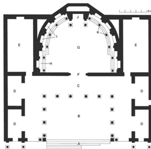
Fig. 4: Plan de la bibliothèque de à Timgad (Numidia) d'après Homer Pfeiffer 1931 planche 16. (Source : Houston, 2014).
