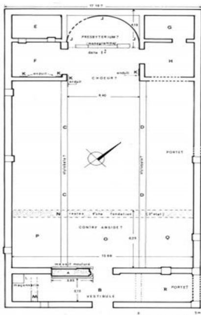
المخطط 02: مخطط البازيليكا المسيحية حسب الباحث
