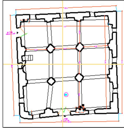
المخطط 01: مخطط الطابق الأرضي للمسجد العتيق. عن: سخري عادل، 2020.
