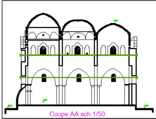
المقطع 01: مقطع AA للمسجد العتيق. عن: سخري عادل، 2020.
