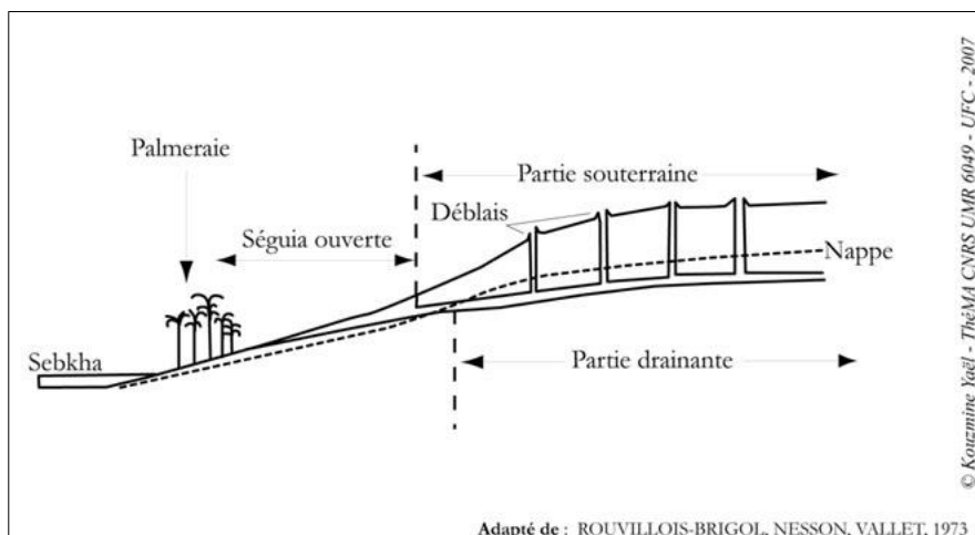
Figure 2 : Croquis de la foggara et de son fonctionnement
