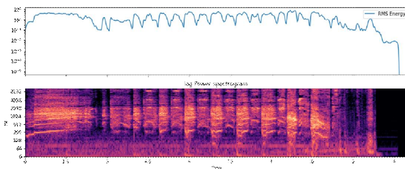
شكل 13: المخطط اللوغارتمي لصوت الحمام
