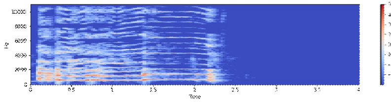
شكل 11: مراتب النغمات الموسيقية لصوت الديك ب
