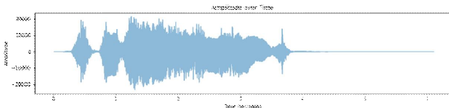
شكل 4: سعة الصوت بدلالة الزمن (الديك أ)
