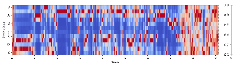
شكل 19: مراتب النغمات الموسيقية لصوت الحمارب
