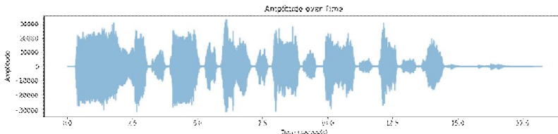
شكل 16: سعة الصوت بدلالة الزمن (الحمار ب)
