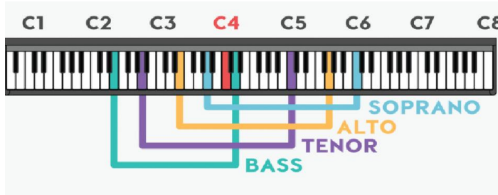
شكل 3: رسم توضيحي للنطاقات الصوتية في علم الموسيقى
