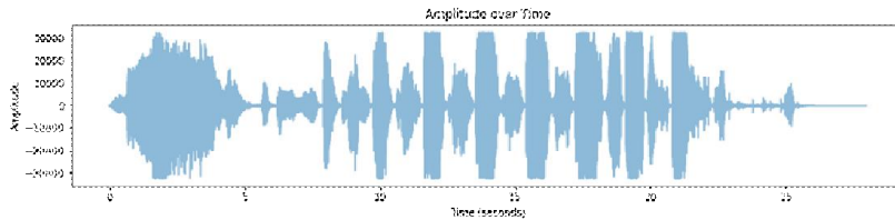
شكل 12: سعة الصوت بدلالة الزمن (الحمار أ)
