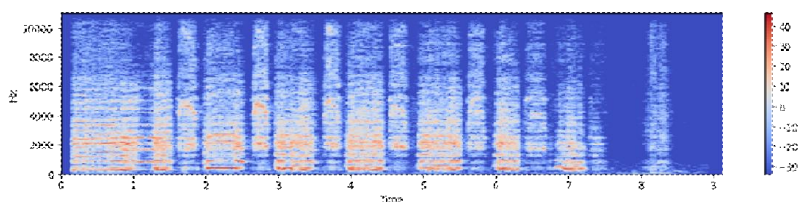
شكل 19: مراتب النغمات الموسيقية لصوت الحمارب
