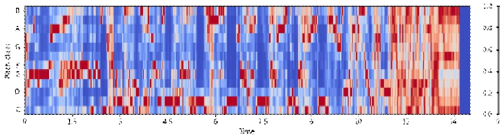
شكل 15: مراتب النغمات الموسيقية لصوت الحمار
