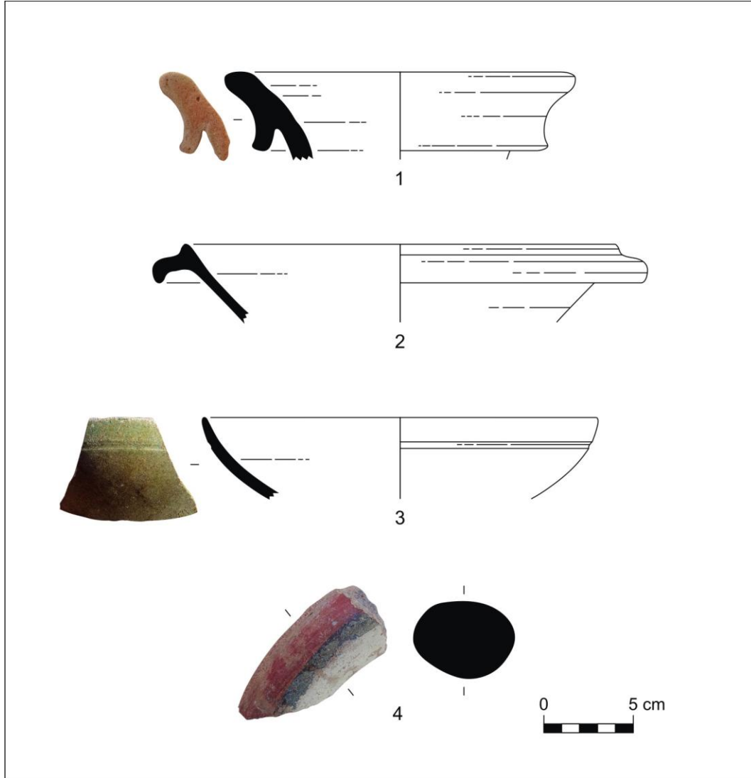
الشكل 01: رسم تقني لمجموعة من القطع الفخارية مع تأريخها، (1- امفورة اسبانية القرن الاول قبل الميلاد- القرن الاول بعد الميلاد)، (2-مهراس سيجيلي القرن 5م)- (3 -صحن عثماني ق16- 18م)- (4-ابريق، ق 19-20). عن: Alejandro Quevedo
