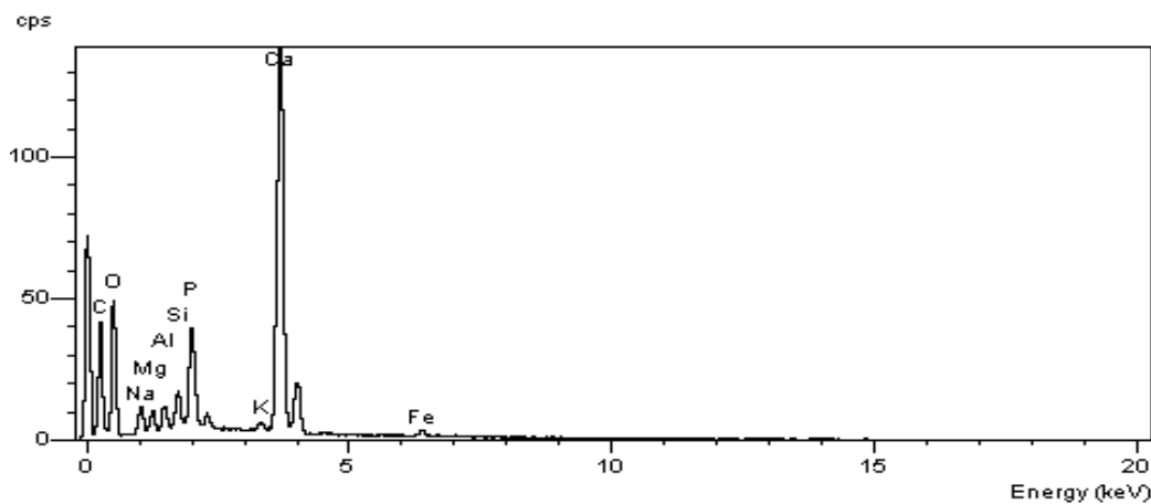
شكل (5): طيف تشتت الطاقة للأشعة اكس (EDX) للكتلة الحية المعالجة
