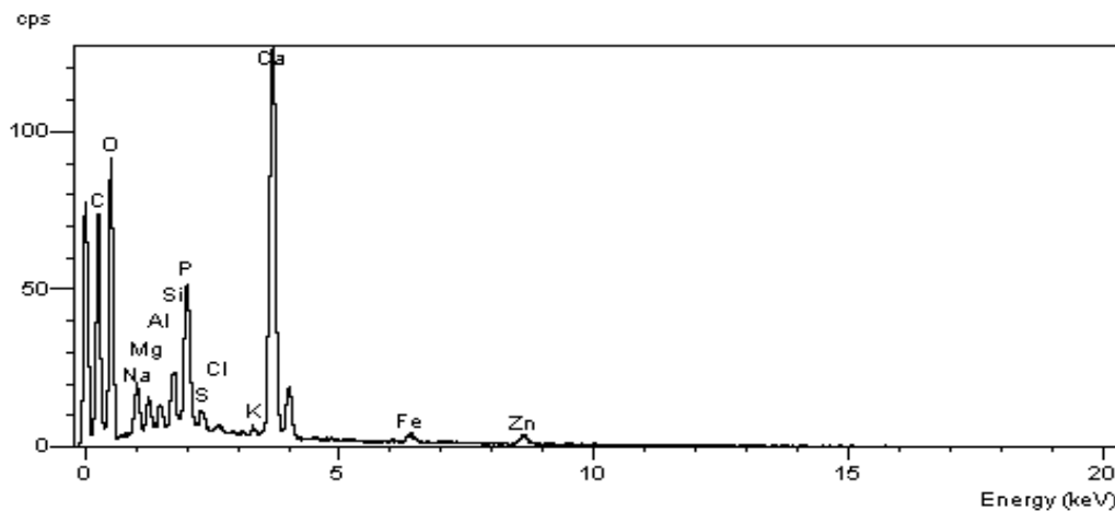
شكل (09): طيف بث الطاقة للأشعة اكس (EDX) للكتلة الحية المعالجة المشبعة بالزنك
