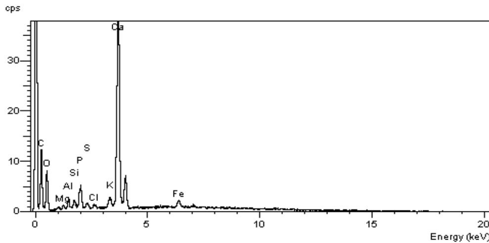
شكل (04): طيف بث الطاقة للأشعة اكس (EDX) للكتلة الحية الخام
