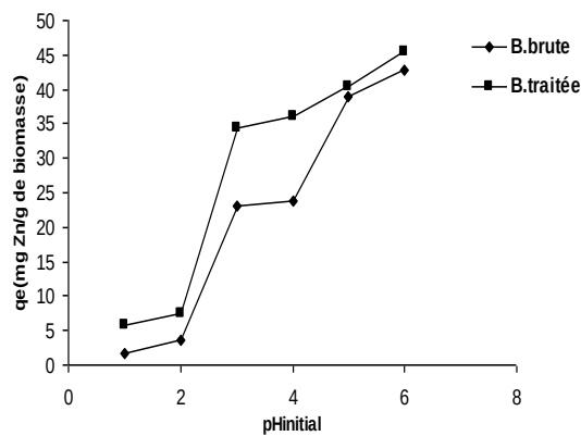
شكل (11): تغير سعة إمتزاز الزنك بدلالة pH الابتدائي للمحلول
