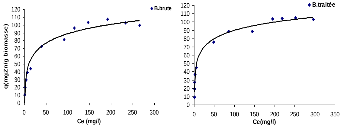
شكل (13): إيزوثرم إمتزاز الزنك من أجل كتلة حية معالجة وخامة
