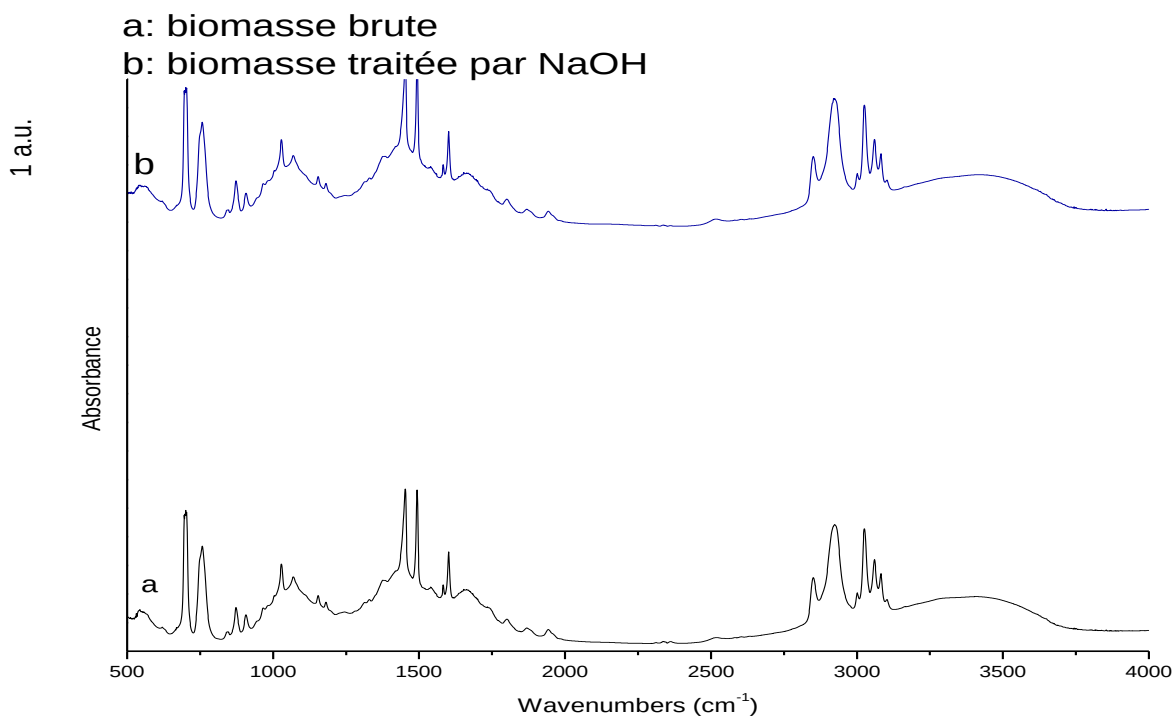
شكل (1): طيف الأشعة تحت الحمراء للكتلة الحية الخام (a) والمعالجة بمحلول هيدروكسيد الصوديوم (b) NaOH
