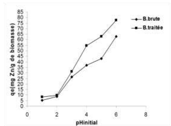
شكل (10): تغير سعة إمتزاز الزنك بدلالة pH الابتدائي للمحلول
