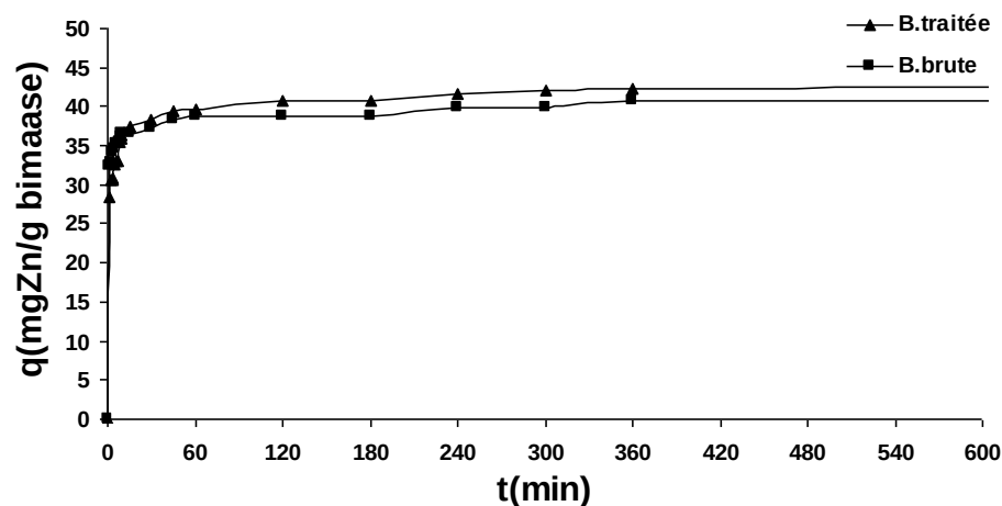
شكل (14): تغير قدرة امتزاز الزنك بدلالة الزمن من أجل كتلة حية خامة و معالجة X = 1 \text{ g/l} , C_0 = 50 \text{ mg/l} , W = 150 \text{ tr/min} , pH = 6 , \theta = 25^\circ\text{C} , t_c = 24\text{h}
