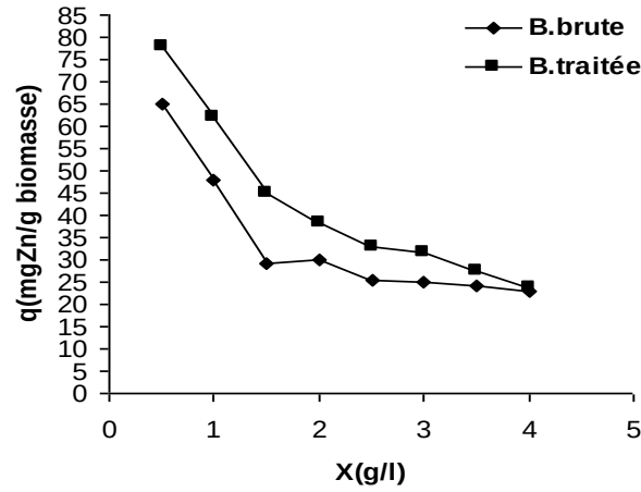
شكل (12): تغير سعة إمتزاز الزنك بدلالة تركيز الكتلة الحية
