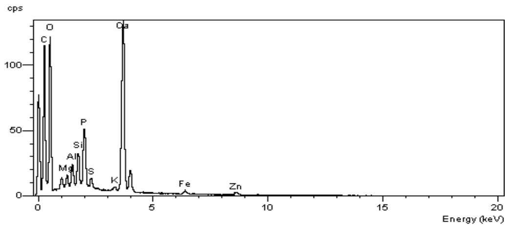
شكل (08): طيف بث الطاقة للأشعة اكس (EDX) للكتلة الحية الخام المشبعة بالزنك
