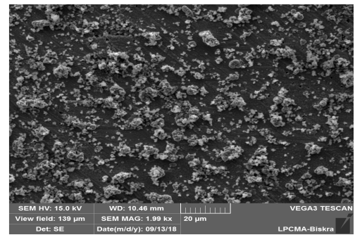
الصورة (2.b) صور المجهر الالكتروني الماسح: DC = 50 % , f = 10 Hz
