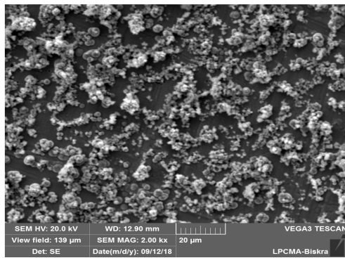
الصورة (2.a) صور المجهر الالكتروني الماسح : DC = 50 % , f = 1 Hz
