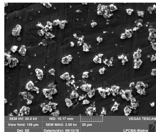
الصورة (2.e) صور المجهر الالكتروني الماسح: DC = 75 % , f = 10 Hz
