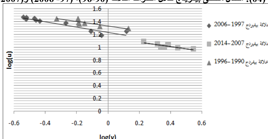
الشكل رقم (04): انتقال منحني بيفريدج خلال الفترات الثلاث (96-90)، (97-2006) و(2007-2014)
