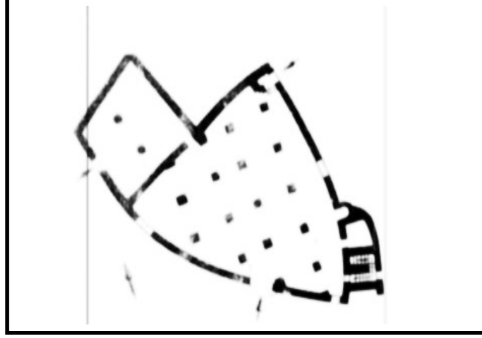
المخطط 01: المسجد العتيق بقصر الشلالة (عن بوحفص سيرات).
