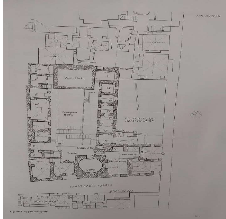
مخطط مسطح الطابق الأول للمدرسة الجوهرية في البلدة القديمة في مدينة القدس
