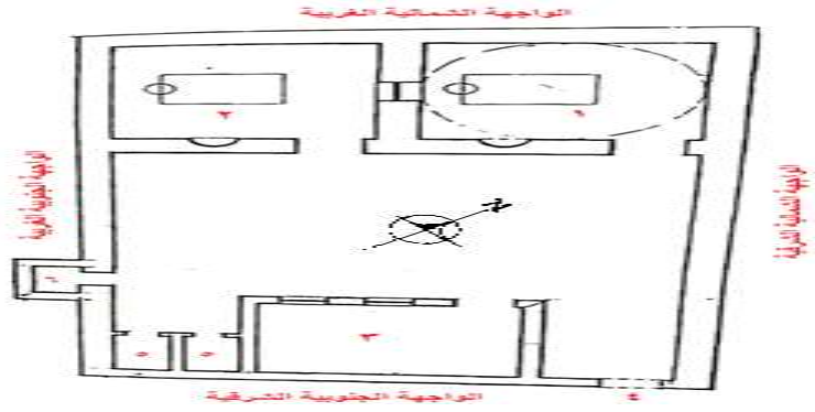
شكل رقم 1، مسقط أفقي للزاوية السنوسية بمدينة القصير- عن عبد الله كامل موسي، القباب الضريحية بمدينة القصير، المرجع السابق، ص 63- بتصرف الباحث.
