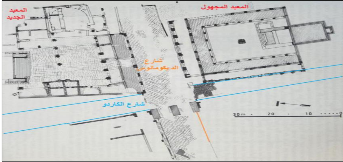
صورة رقم 4: مخطط تقاطع شارع الديكومانوس مع الكاردو (مدينة تيبازة الاثرية)
