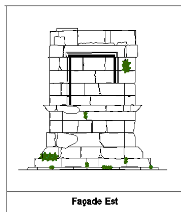
Plan 7. Façade Est
