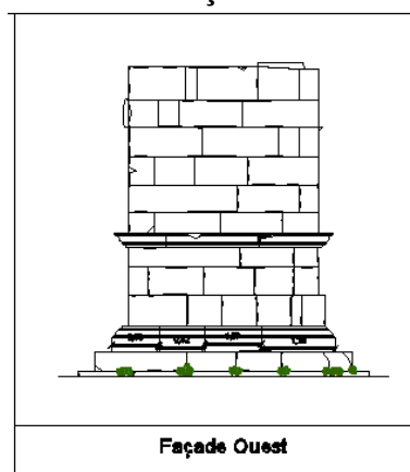
Plan 6. Façade Ouest
