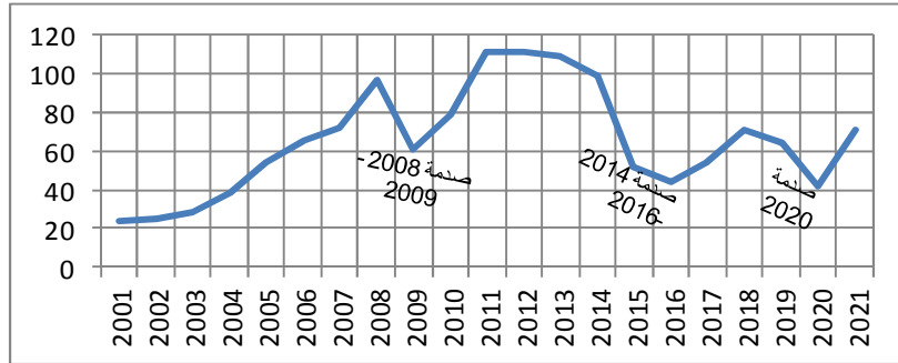
الشكل 01: تطور متوسط أسعار النفط السنوي خلال الفترة 2001-2021
