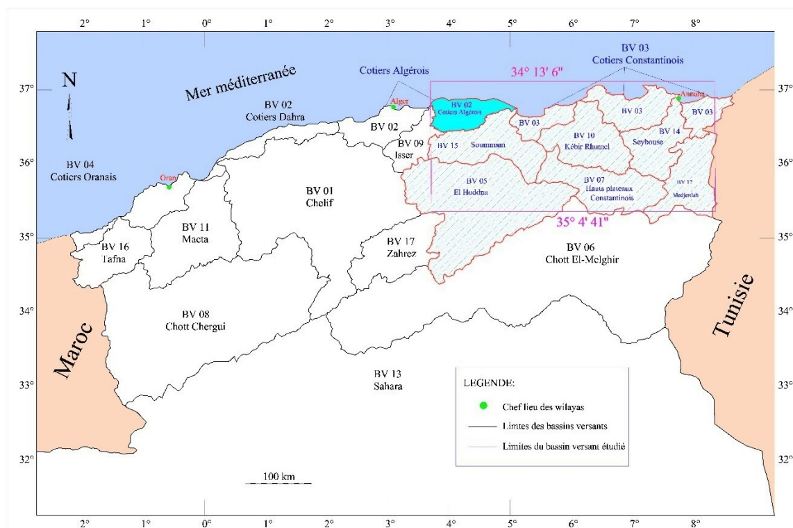
Figure 01 : Carte des Bassins versants et les limites de l'Agence Nationale des bassins hydrographiques.
