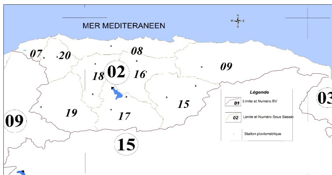
Figure 02: Répartition des stations pluviométriques dans le Nord-Est d'Algérie.
