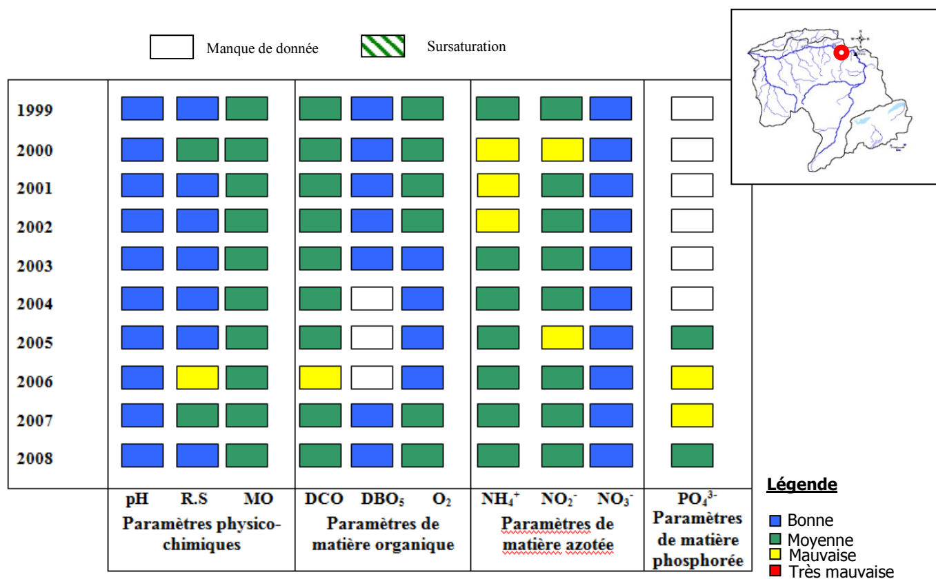
Figure 4 : Fiche de Qualité moyenne annuelle des eaux de barrage Harreza (1999-2008)
