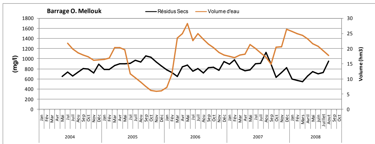
Figure 6 : évolution des résidus secs et du volume d'eau dans les barrages.
