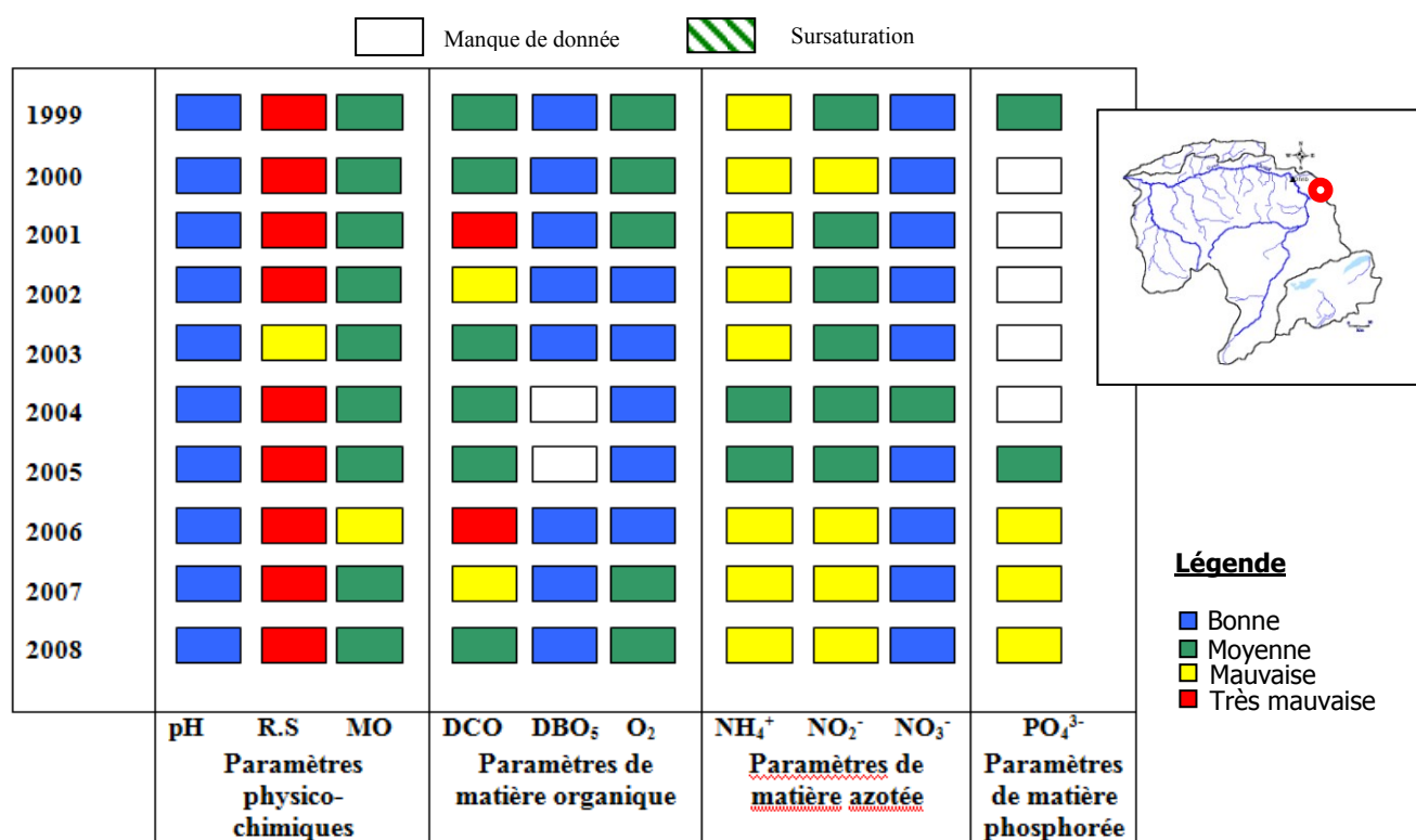
Figure 2 : Fiche de Qualité moyenne annuelle des eaux de barrage Ghib (1999-2008)
