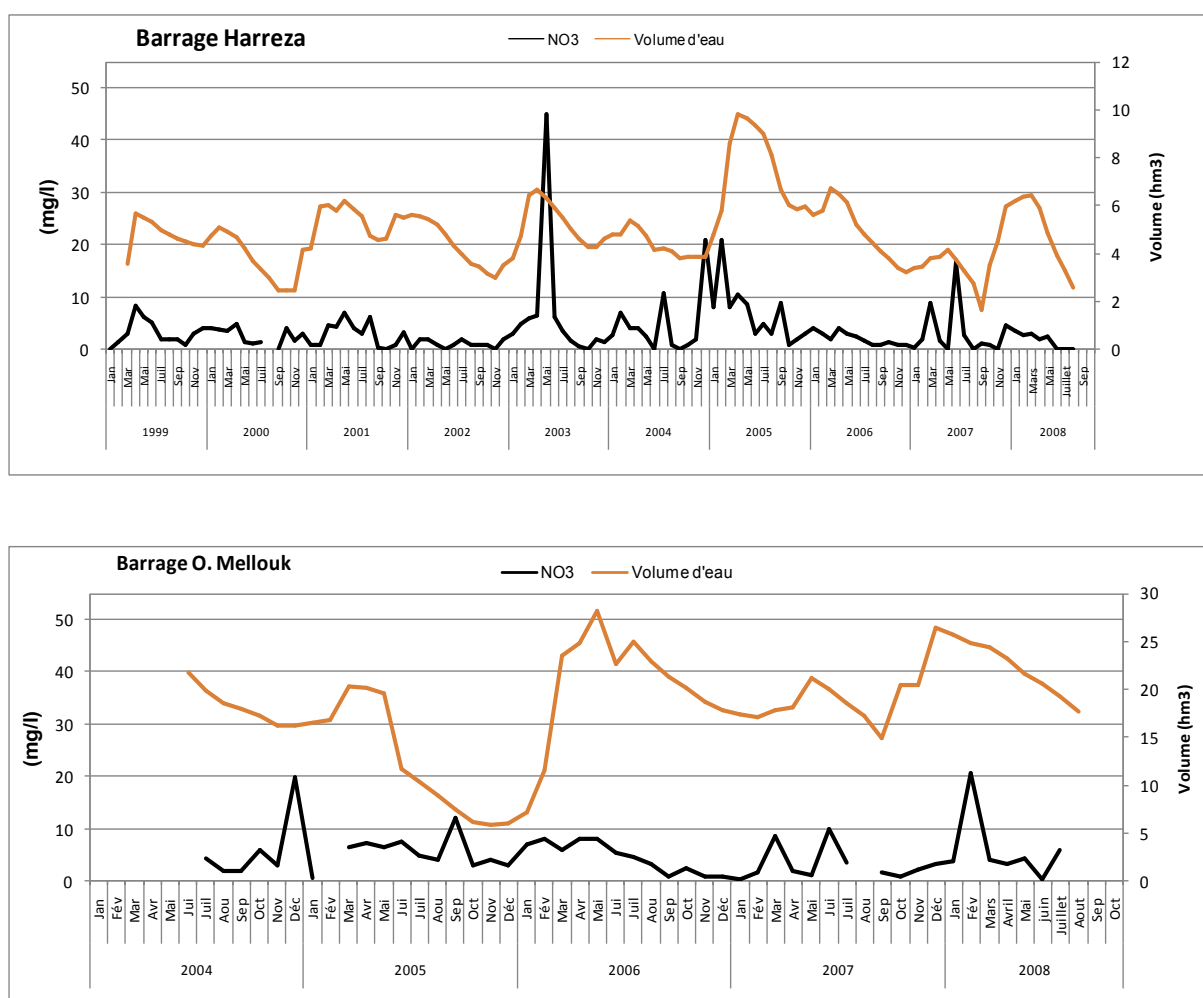
Figure 8 : évolution des \text{NO}_3^- et du volume d'eau dans les barrages.
