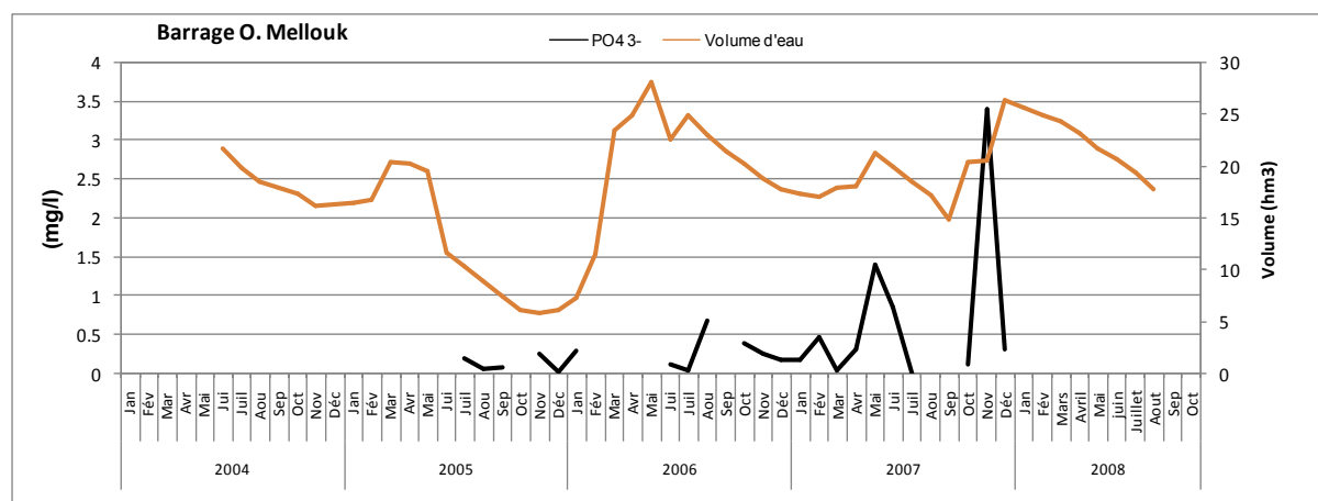
Figure 9 : Évolution des \text{PO}_4^{3-} et du volume d'eau dans les barrages.
