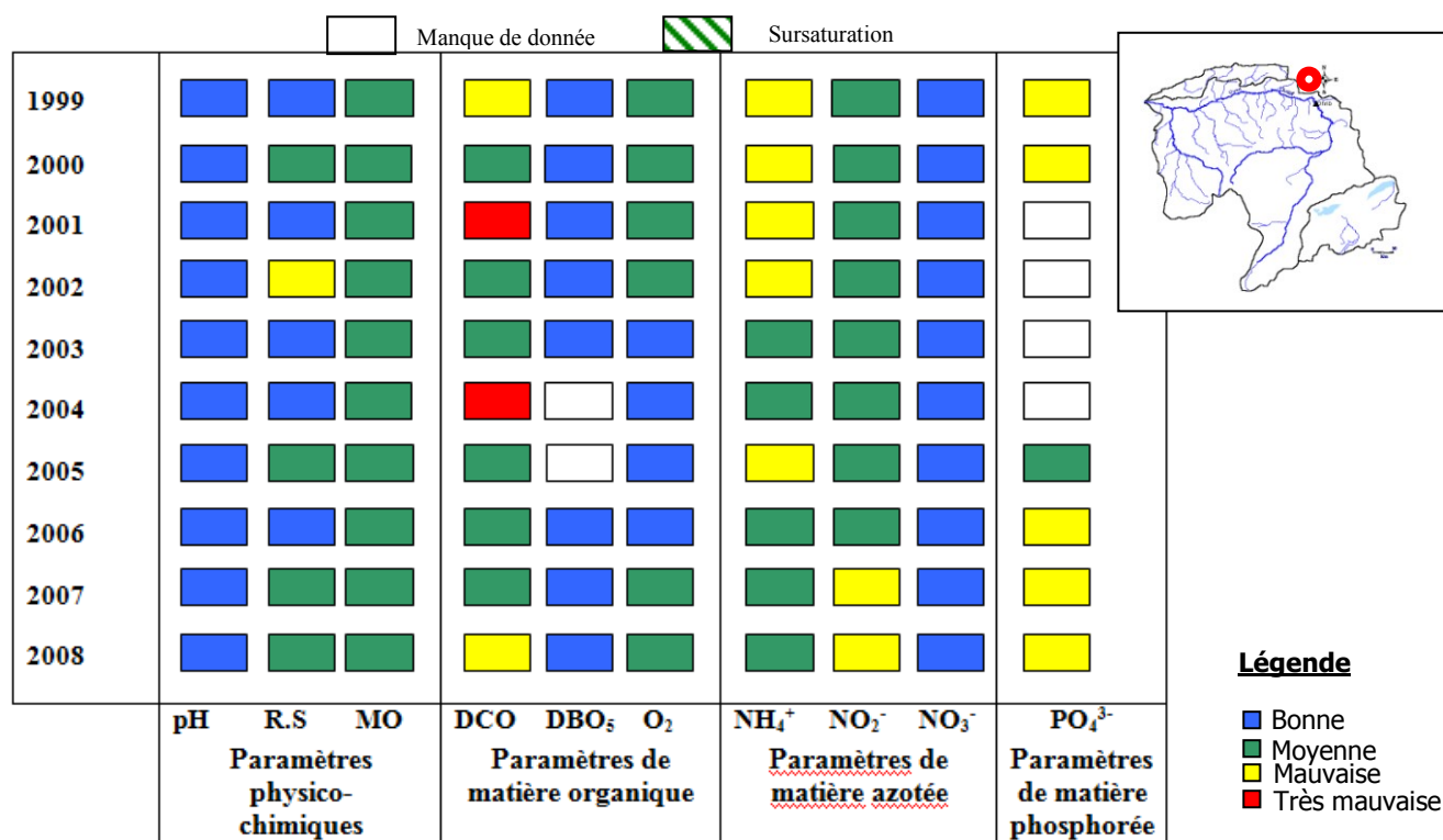
Figure 3 : Fiche de Qualité moyenne annuelle des eaux de barrage Deurdeur (1999-2008)
