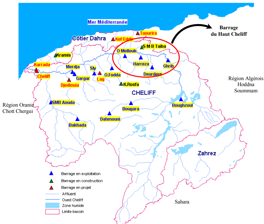
Figure 2: Répartition des barrages dans le bassin du Haut Cheliff.
