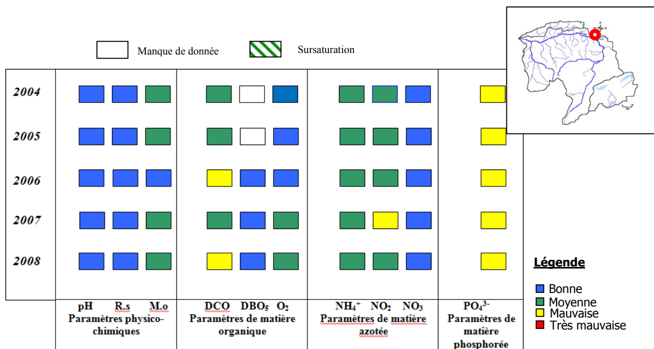
Figure 5 : Fiche de Qualité moyenne annuelle des eaux de barrage O. Mellouk (2004-2008)
