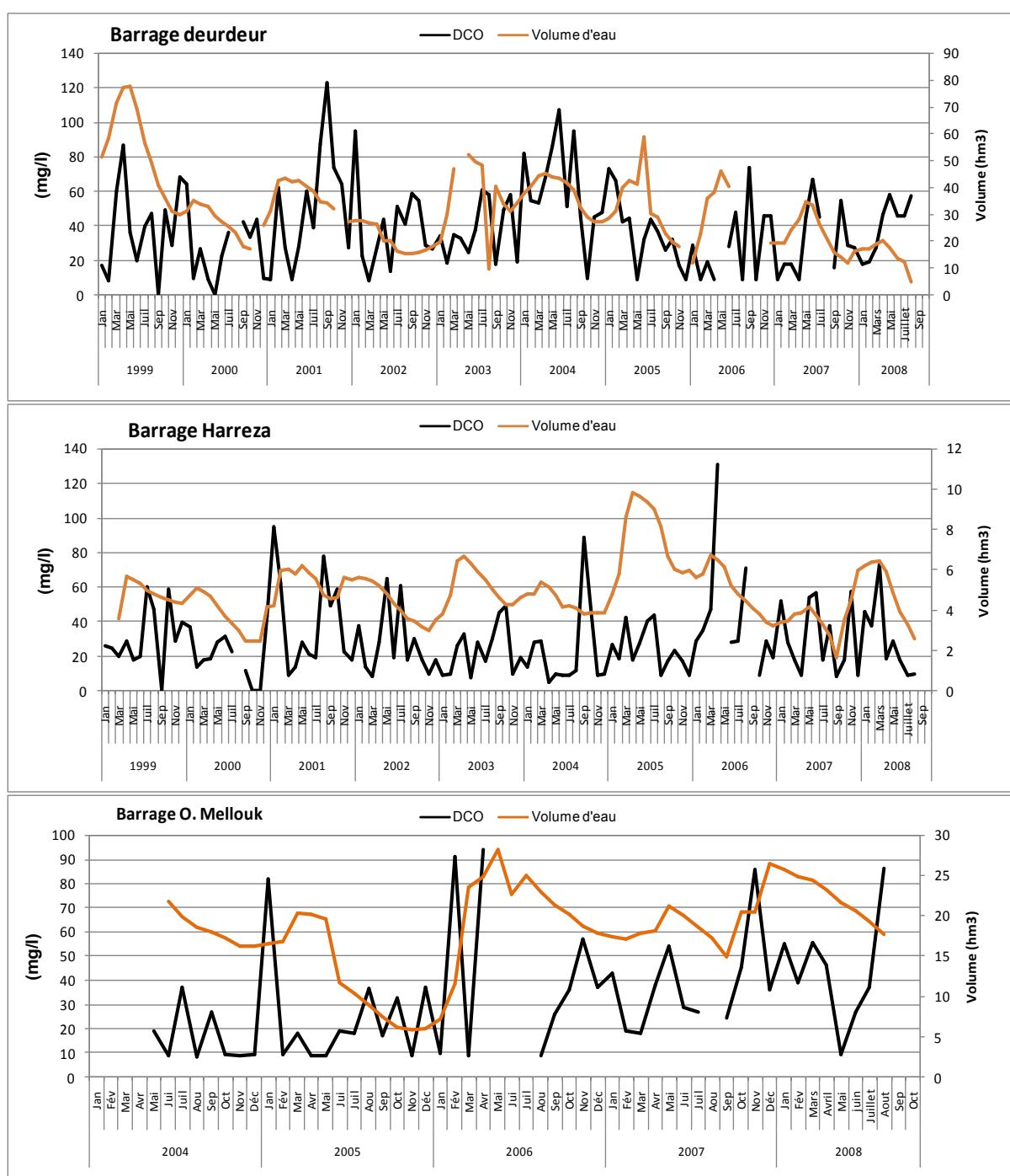
Figure 7 : évolution des DCO et du volume d'eau dans les barrages.
