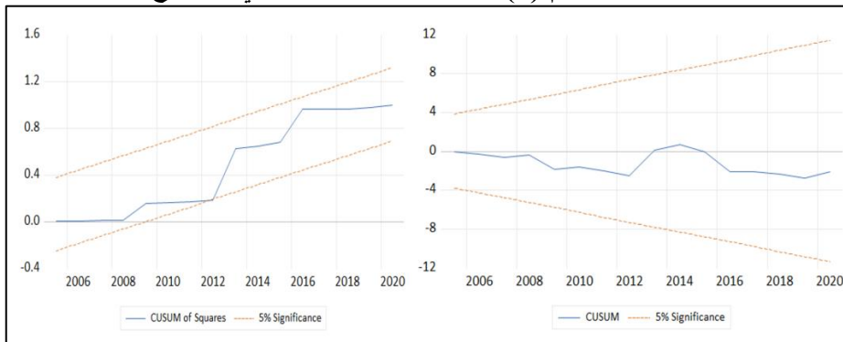
شكل رقم (3): اختبار الاستقرار الهيكلي للنموذج
