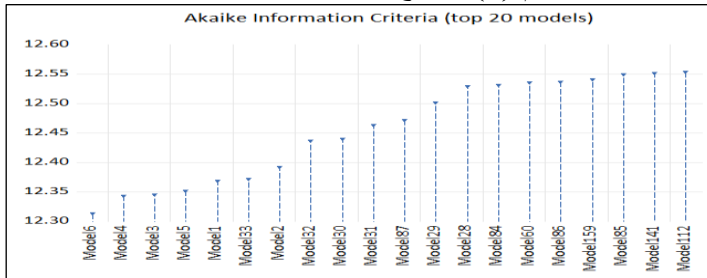
شكل رقم (1): نتائج اختبار فترة الإبطاء المثلى
