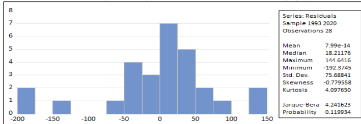
شكل رقم (2): اختبار التوزيع الطبيعي لبواقي النموذج المقدر
