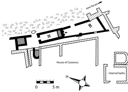
المخطط 09: الحمّامات الصّغرى (الشمالية الشرقية) لمنزل كاستوريوس. عن: SADI, M., 2016, p. 131.
