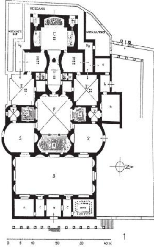
المخطط 01: مخطط الحمامات الكبرى الجنوبية بمدينة كويكول. عن: THEBERT, Y., 2003, pl. LXXV.
