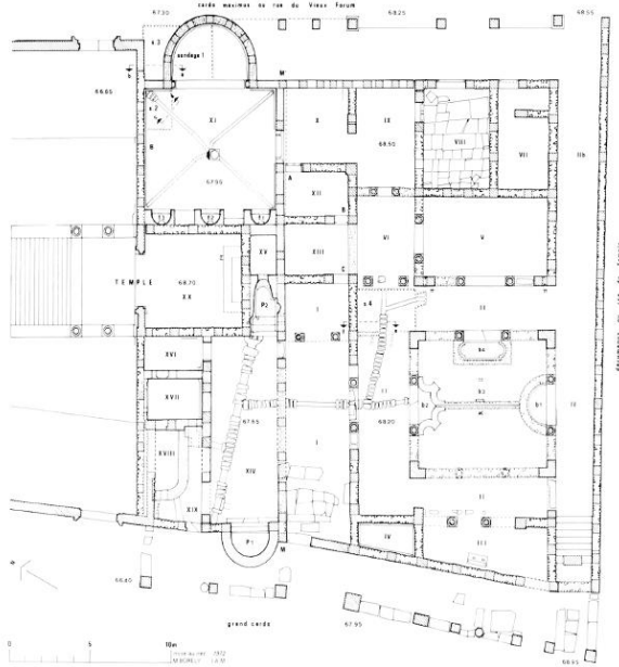
المخطط 07: منزل الحمار بمدينة كويكول. عن:
