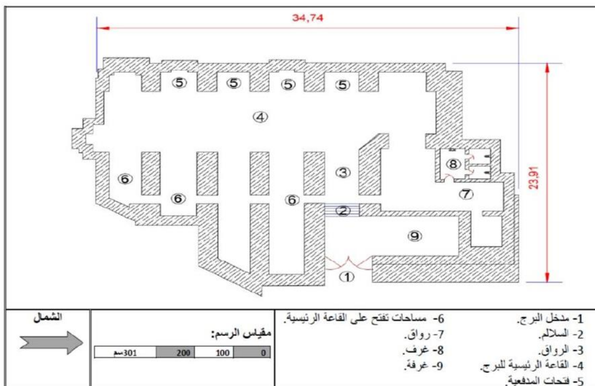
المخطط 01: برج مابين. عن: عمل الباحثين.
