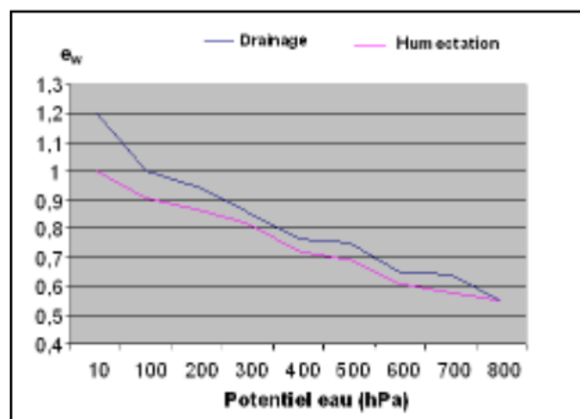
Figure 1 : Courbes d'hystérésis des agrégats millimétriques
