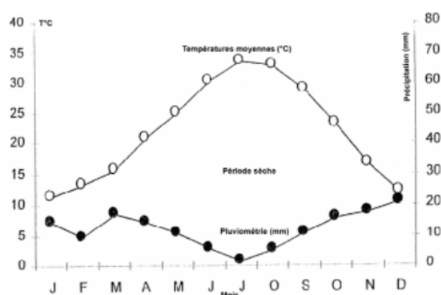
Figure 3b : Diagramme ombrothermique pour la période allant de 1985 – 2001 de la région de Biskra
