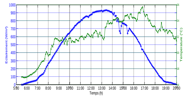
Figure 2. Évolution au cours du temps de l'éclairement solaire pendant la journée d'essai.
