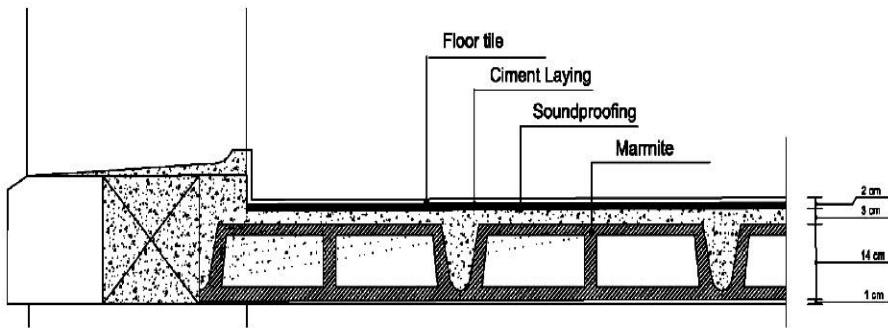
Fig. 10: Le plancher Pouillon
