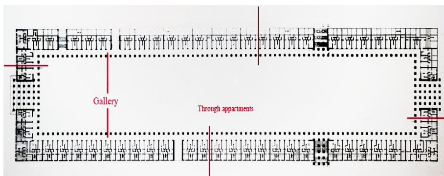
Fig. 6: les appartements traversant de Climat de France
