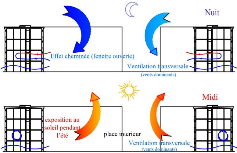
Fig. 8: Ventilation naturelle (transversale et effet cheminée) à Climat de France
