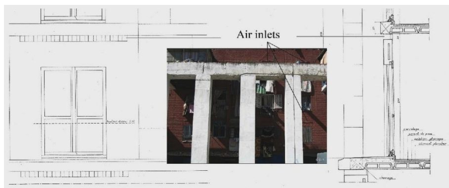
Fig. 7: Les amenées d'air des fenêtres de façade de Climat de France
