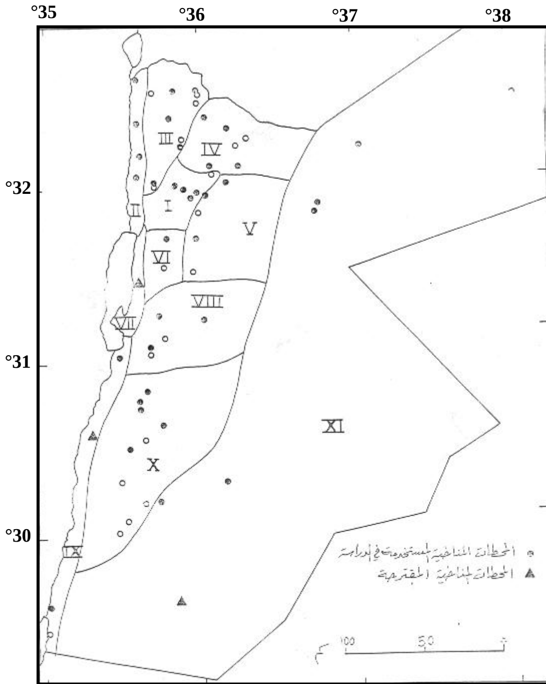
شكل 4. المناطق المناخية المتشابهة وفق درجة الحرارة الصغرى
