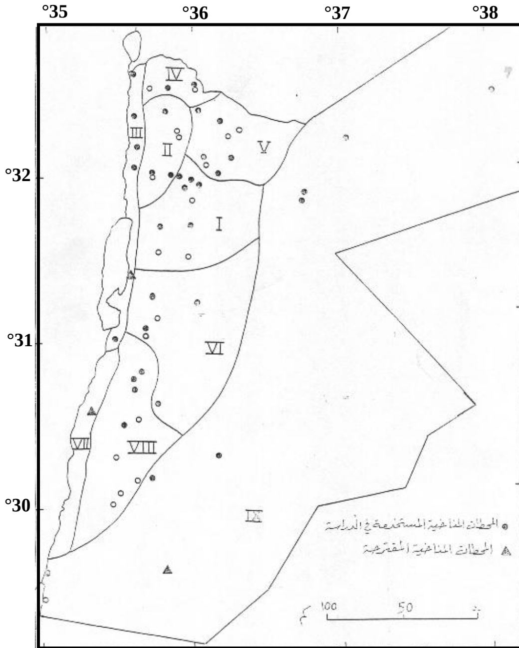
شكل 3. المناطق المناخية المتشابهة وفق درجة الحرارة العظمى
