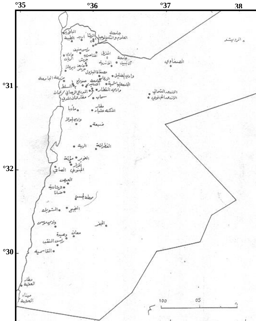
شكل 1. المحطات المناخية في الأردن
