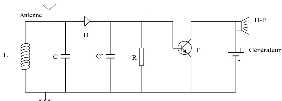
Schéma simplifié du poste récepteur
