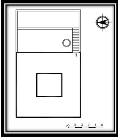
1- سلم. المخطط رقم 06: مخطط سطح منزل عبيد - عن الطالب-
