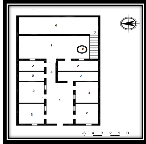
1- صحن. 2- غرفة. 3- مطبخ. 4- رواق. المخطط رقم 05: مخطط الطابق الأرضي لمنزل عبيد - عن الطالب-
