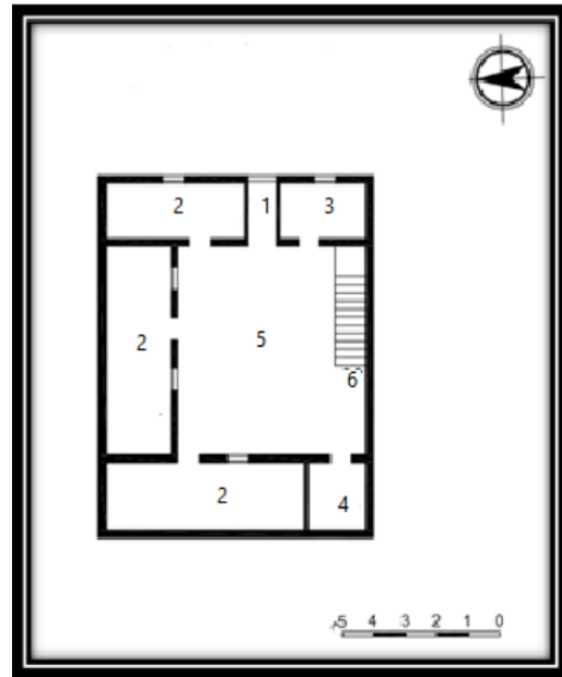
1- سقيفة. 2- غرفة. 3- مطبخ. 4- مرحاض. 5- صحن. 6- سلم. المخطط رقم 03: مخطط الطابق الأرضي لمنزل شامي - عن الطالب-
