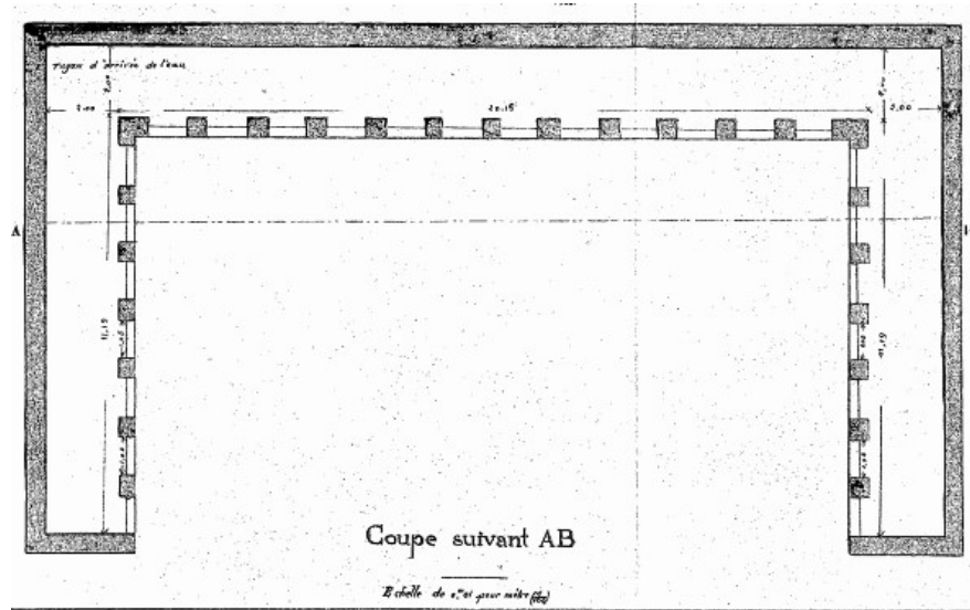
الشكل رقم 04: مقطع أفقي لخزان حديقة رفاوي. المرجع: Ibid
