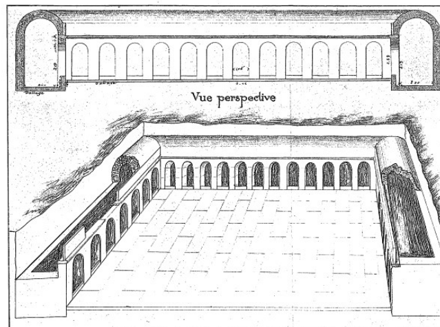
الشكل رقم 03: مخطط ثلاثي الأبعاد لخزان حديقة رفاوي. المرجع:
