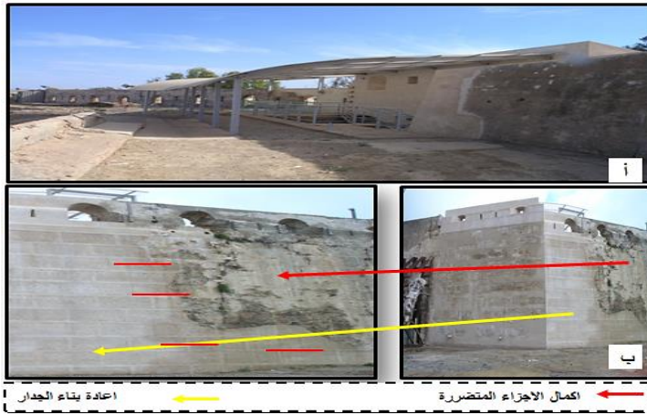
صورة رقم (06) : شكل الجدار بعد عملية الترميم داخليا وخارجيا
