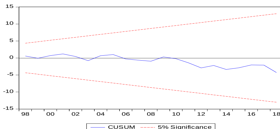
الشكل رقم(1): نتائج اختبار المجموع التراكمي للبواقي ( Cusum Test ) .
