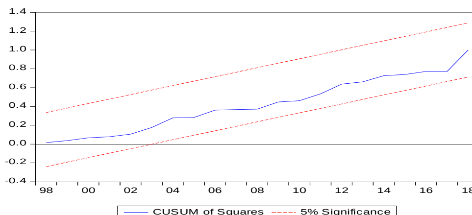
الشكل رقم(2): نتائج اختبار المجموع التراكمي لمربعات البواقي (Cusum of Squares) .
