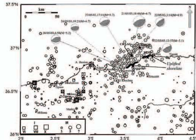
Figure 2: Répartition des répliques et mécanismes au foyer des chocs principaux liés au séisme du 21 mai 2003 (Ayadi et al., 2003 ; les étoiles représentent les différentes localisations des épicentres du séisme, voir aussi Figure 5). On peut noter la répartition oblique à la côte des répliques et la remarquable similarité des solutions focales
