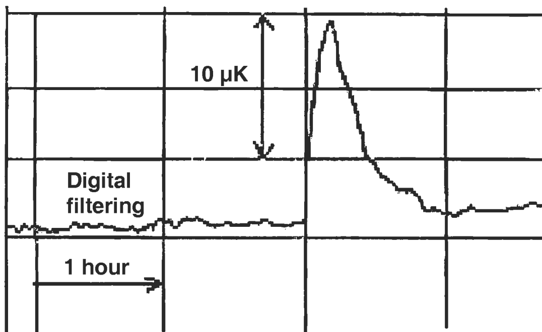
Fig. 5 Enregistrement à Walferdange, par le thermomètre équipé d'un pont de thermistances, d'une variation de température de 13 \mu K. Le site d'installation est le fond d'un forage d'un mètre de profondeur dans le gypse de la mine en bout de galerie.
