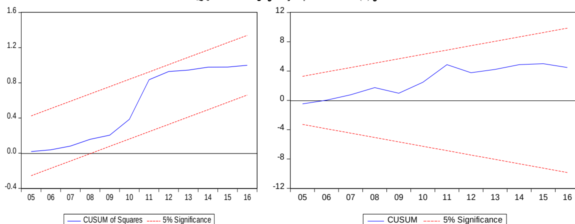
الشكل (2): لأشكال البيانية لاختبارات كل من CUSUM و CUSUMSQ.
