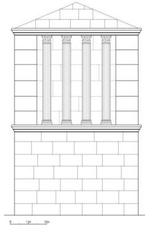
الشكل 03: الواجهة الأمامية لضريح مورسط.
