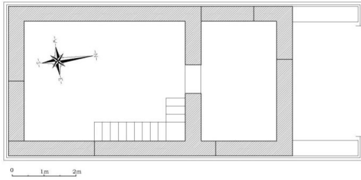
مخطط 02: مقطع أفقي لضريح زانا في مستوى الطابق الأرضي.
