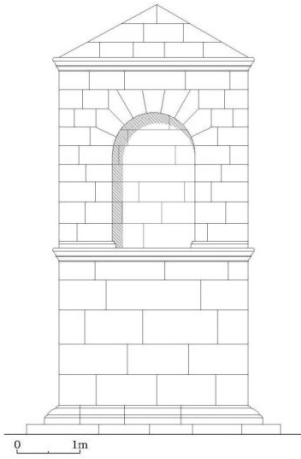
الشكل 04: الواجهة الأمامية لضريح رأس العيون.
