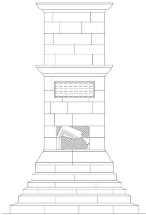
الشكل 09: الواجهة الأمامية لضريح صومعة الخناق.
