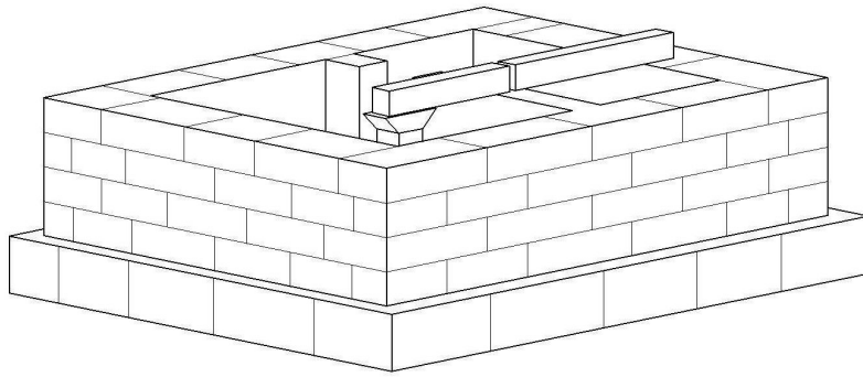
الشكل 05: منظر ثلاثي الأبعاد لضريح فليكس بولكس (كيسا).
