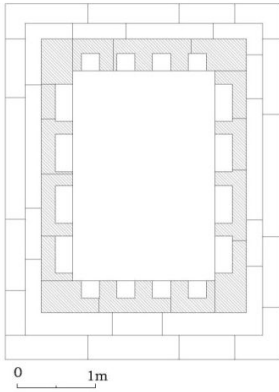
مخطط 01: مقطع أفقي لضريح رأس العيون.
