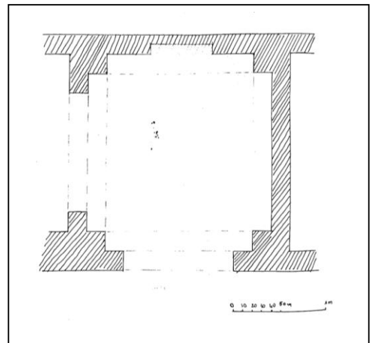
لوحة 2: نماذج لمخططات مساكن مدينة سدراته (عن حملاوي)
