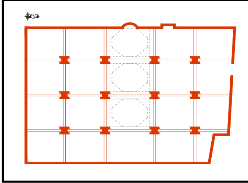
المخطط 03: بيت صلاة جامع قسبة بجاية ( عمل الباحثين ).
