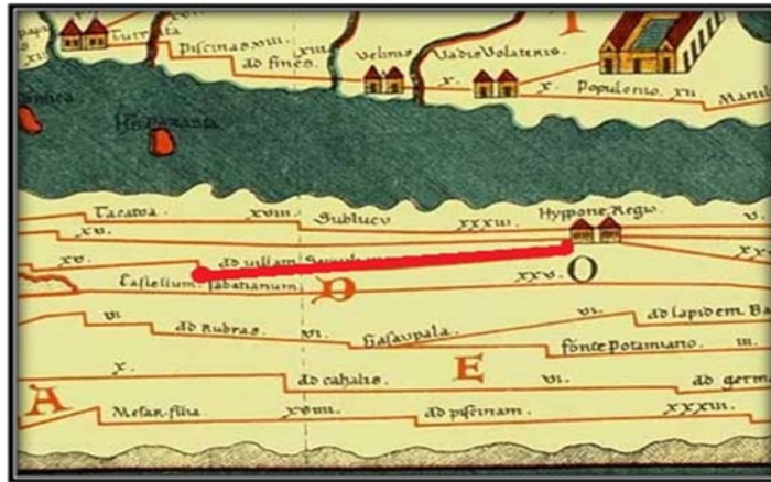
الشكل رقم 2: خريطة بوتينجر
