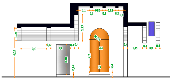
مخطط رقم (03)/ ساباط سوق العصر- مقطع 1.
