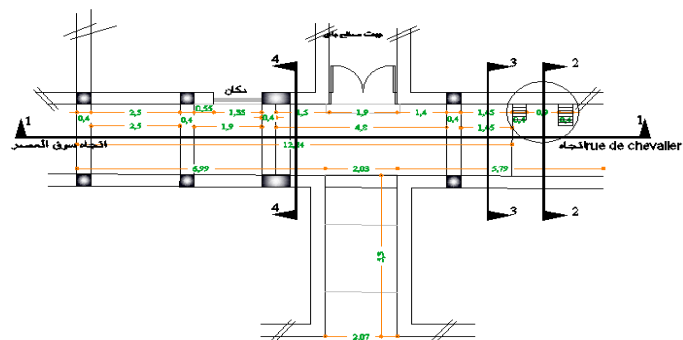
مخطط رقم (02)/ ساباط سوق العصر.
