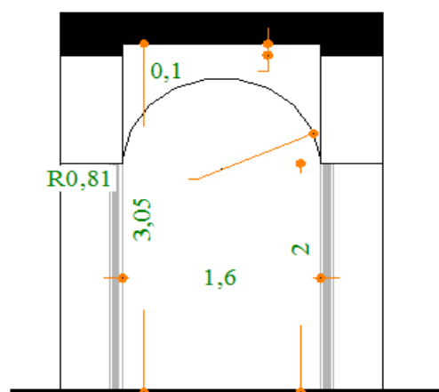
مخطط رقم (06)/ ساباط الكورة- مقطع 2.
