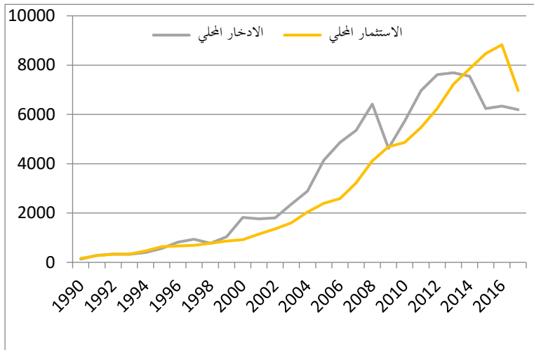
الشكل (2): العلاقة بين الادخار المحلي والاستثمار المحلي في الجزائر. الوحدة: (مليار دج)
