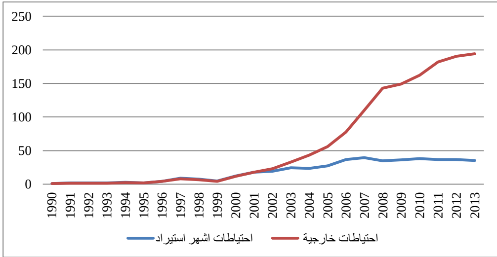
الشكل رقم 02: تطور احتياطات الصرف الاجنبي و معدل التغطية خلال الفترة 1990-2013
