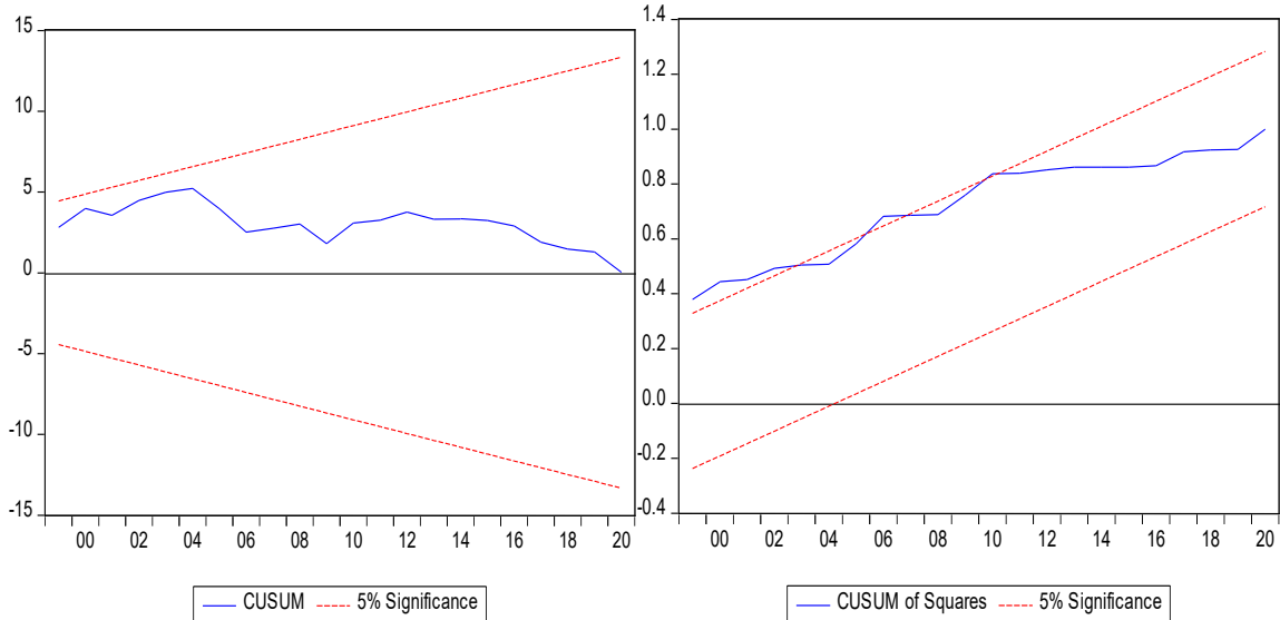
الشكل(01): اختبار المجموع التراكمي للبواقي والمجموع التراكمي لمربعات البواقي المعاودة
