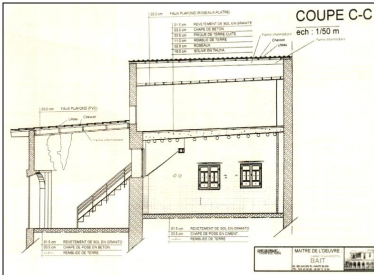
Fig. 5 - Vue en coupe. Côte ouest de la salle de prière.
