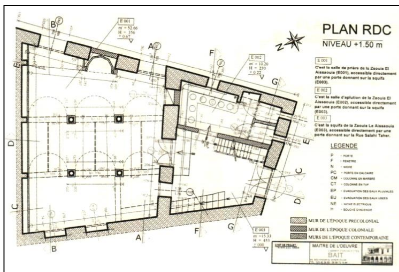
Fig. 2 – Vue en plan de la zaouïa.
