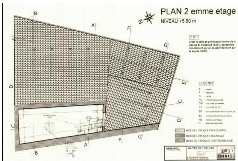
Fig. 3 – Vue en plan de l'étage et de la toiture.
