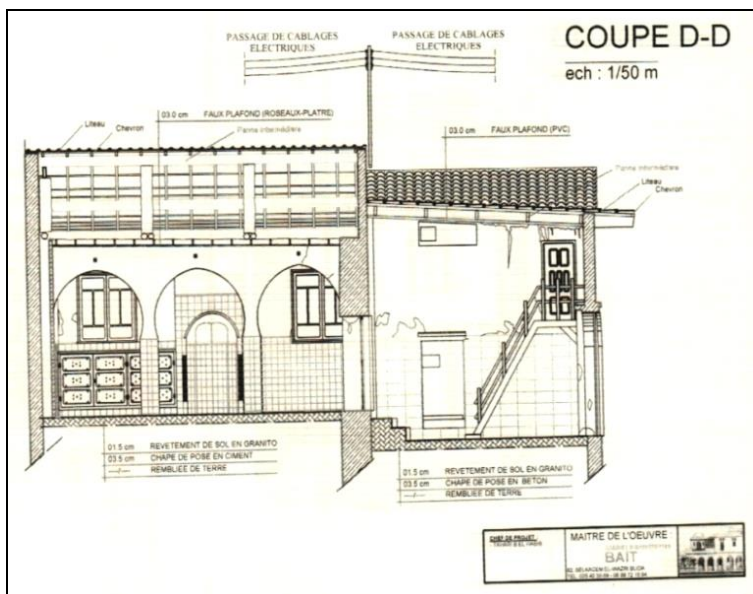
Fig. 4 - Vue en coupe. Côté du mihrab.
