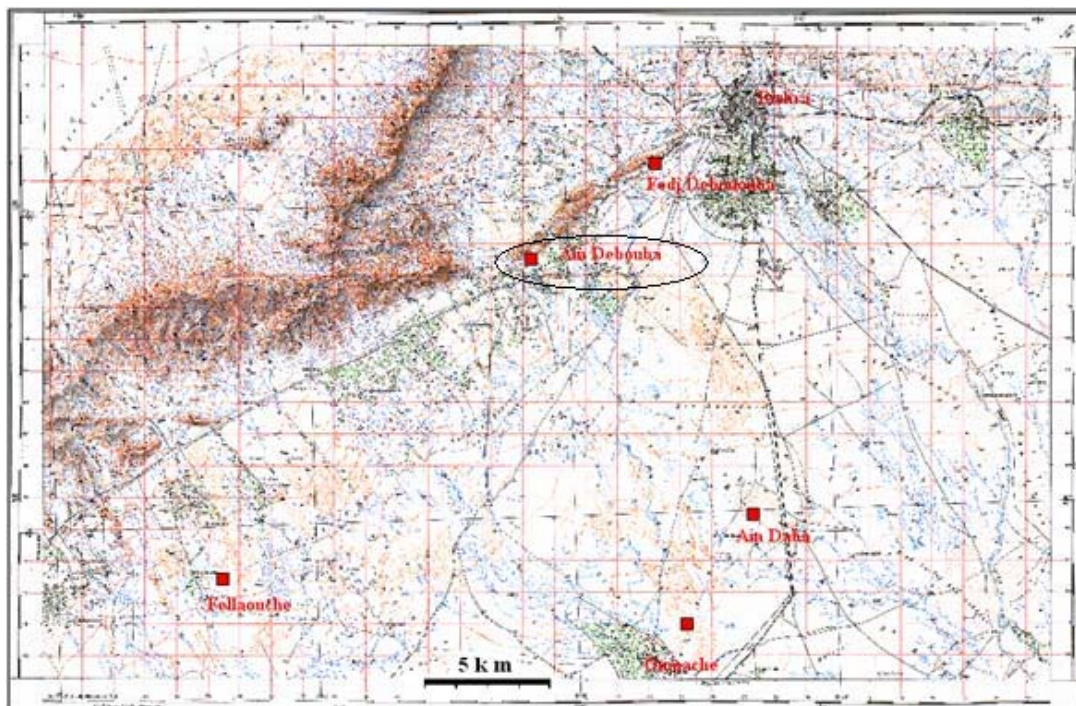
Figure 2: Situation géographique de la station d'étude (N : 34°48' 47,9'', E: 05°39'16,7'', Alt: 122 m)
