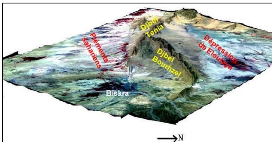
Figure 1 : Modèle numérique du terrain de la région d'étude (BENAZOUZ et al., 2007)
