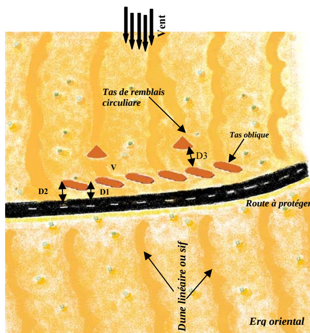
Fig. 7. Dispositif du tas de remblais orienté obliquement par rapport à la route en plus des tas sous forme circulaire(ELMETHANA)
